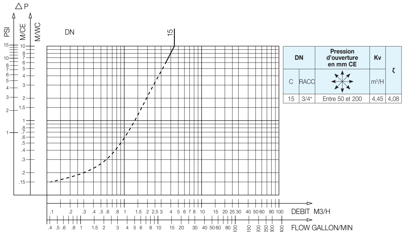
EA 251S - Abaque des pertes de charge
