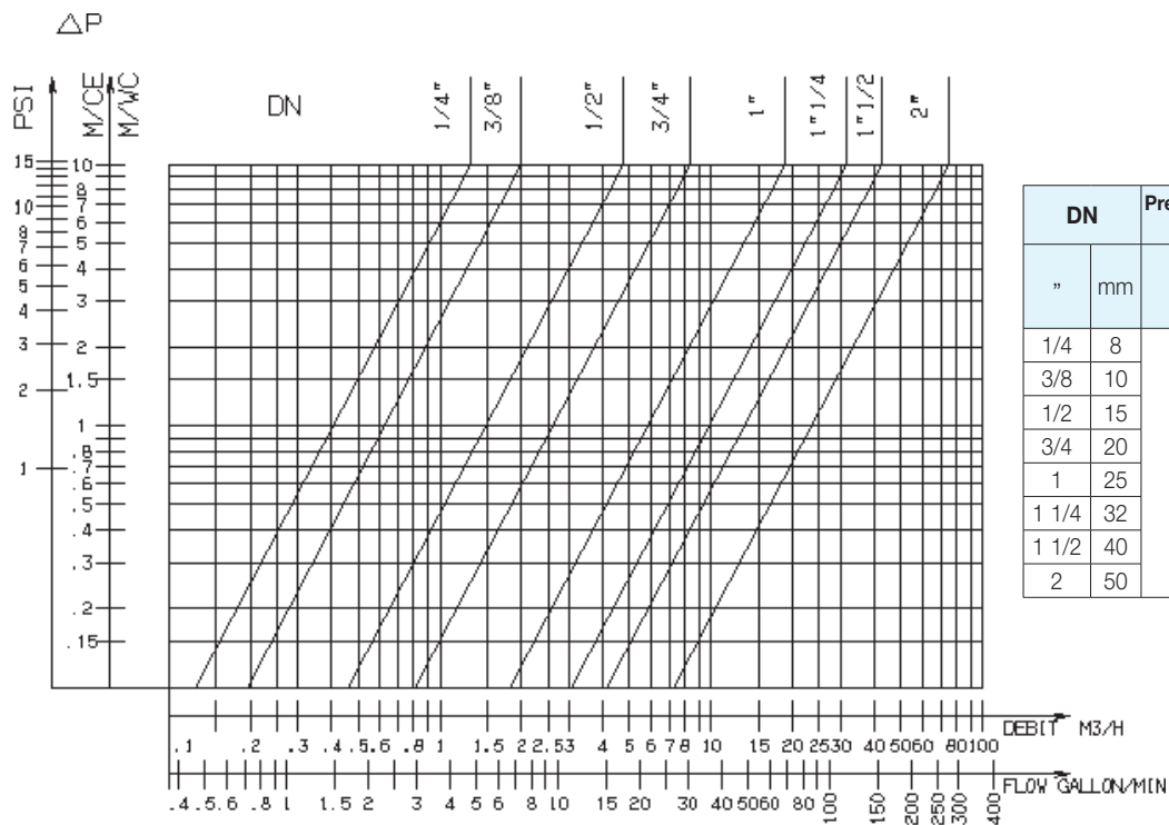
233X - Abaque des pertes de charge
